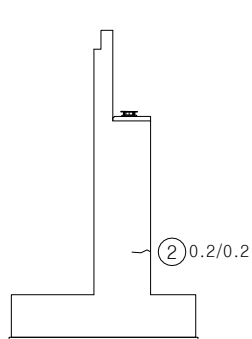
좌측면
